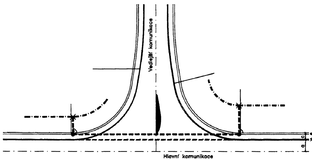
OBR.1 - ÚROVNŮVÁ KŘÍŽOVATKA BEZ SMĚROVACÍCH OSTRŮVKŮ NA VEDLEJŠÍ KOMUNIKACI NEBO SE SMĚROVACÍMI OSTRŮVKY MIMO VOLNOU ŠÍŘKU HLAVNÍ KOMUNIKACE
